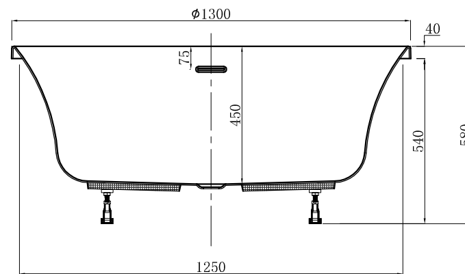
截面 F-F
