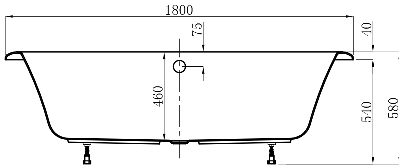
截面 F-F
