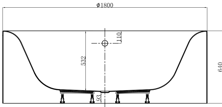
剖面图 A-A
