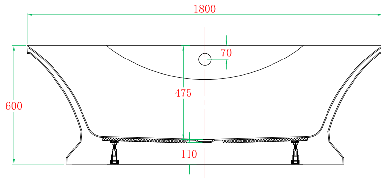
剖视图 A-A
