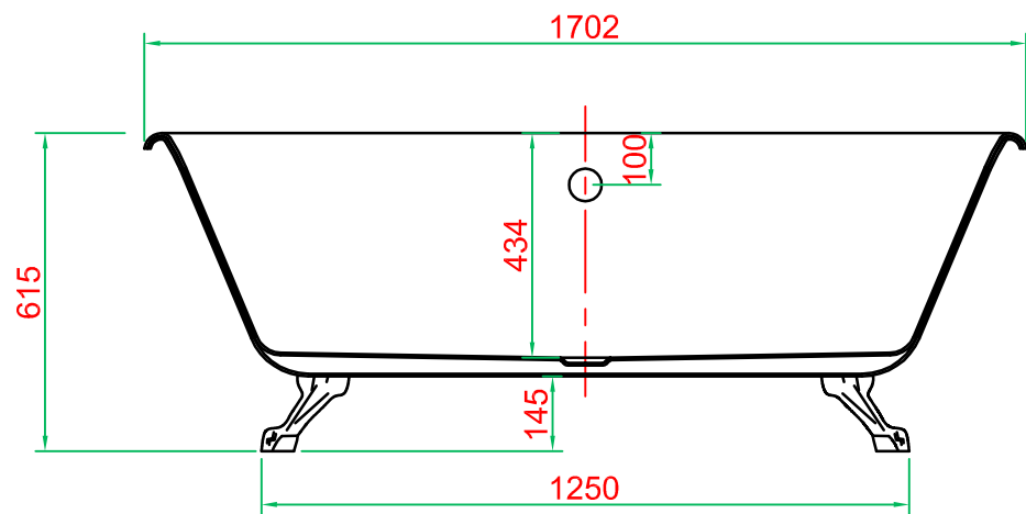
剖视图 A-A
