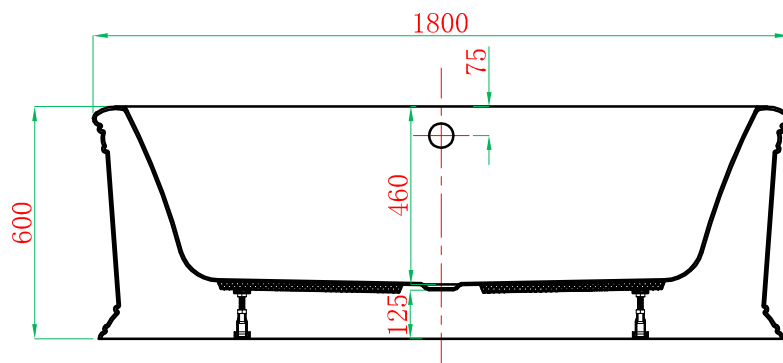
截面 F-F
