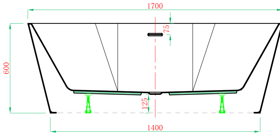
截面 F-F
