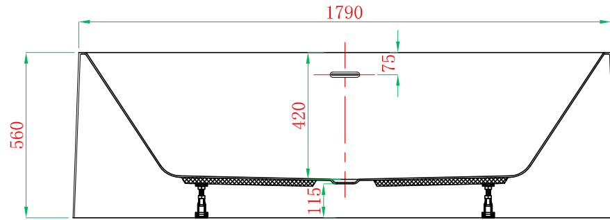
剖视图 F-F
