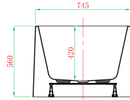
剖视图 G-G
