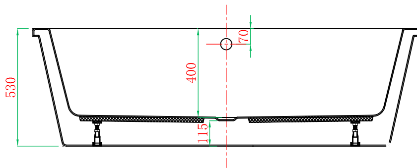
截面 F-F
