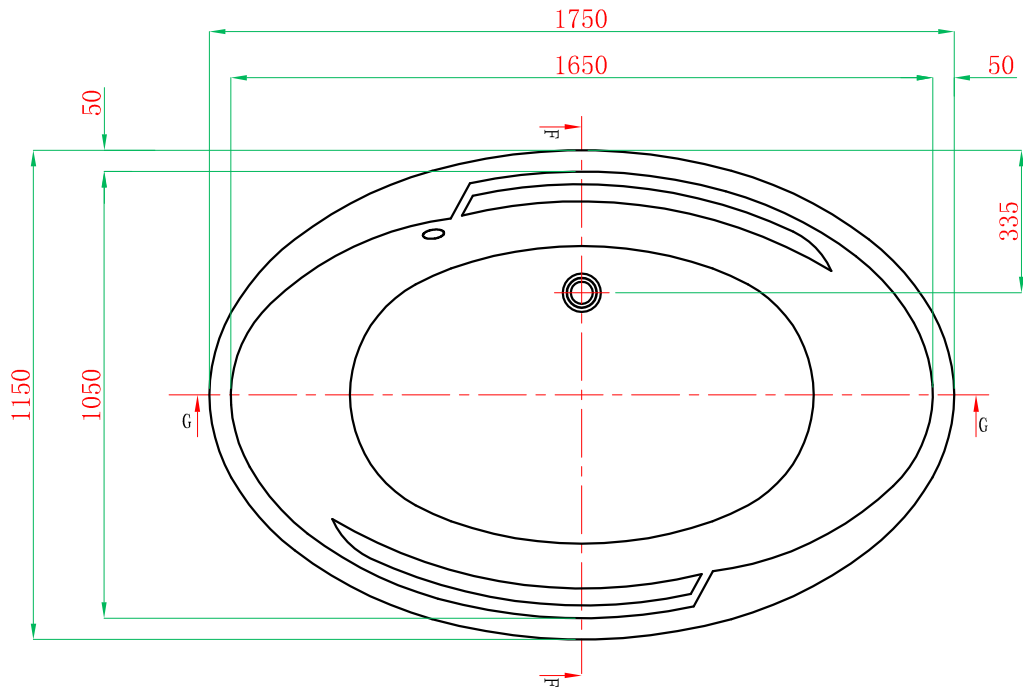
主视图
