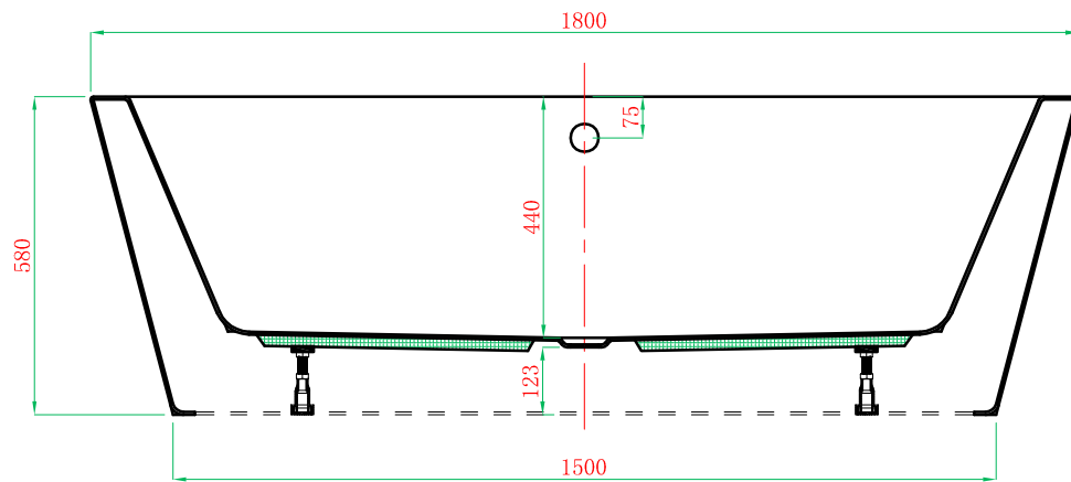
Section A-A
