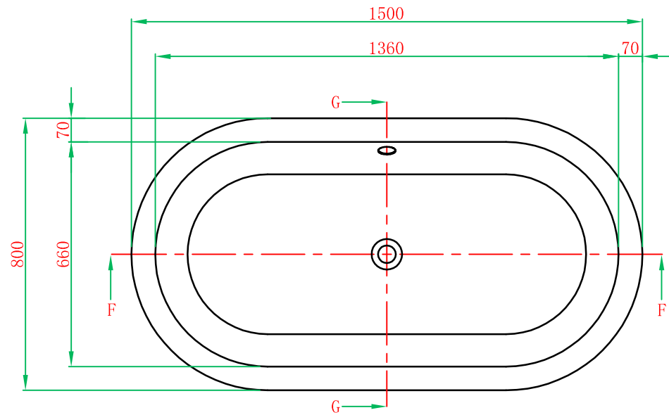
主视图
