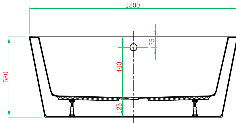
主视图
