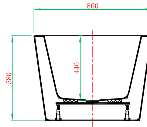
G-G 剖面图
