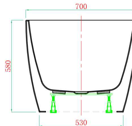
截面 G-G
