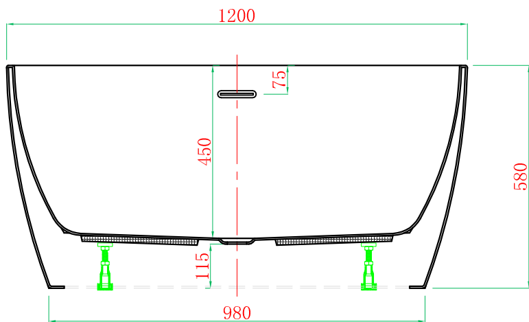
截面 F-F
