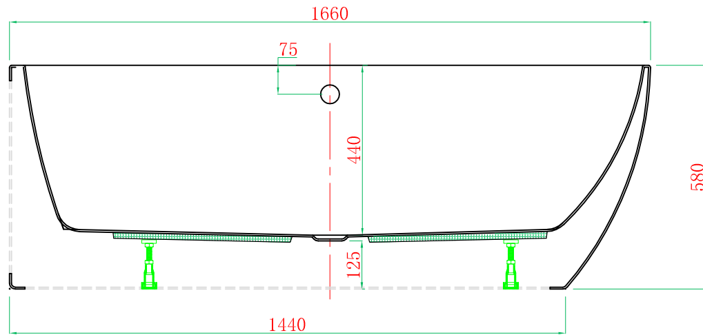
截面 F-F
