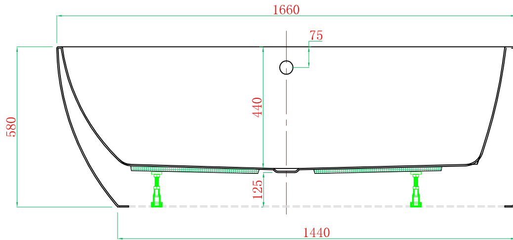
截面 F-F
