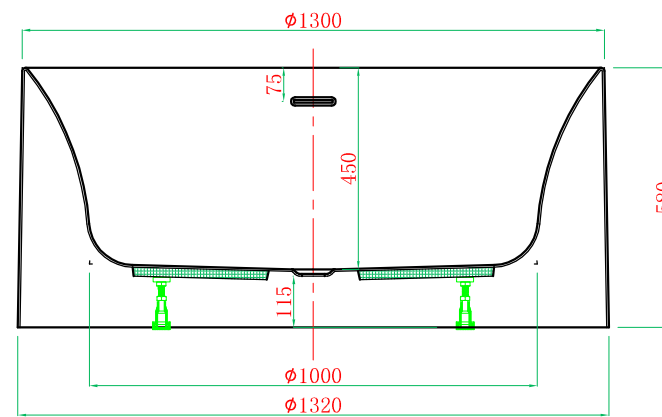
截面 F-F
