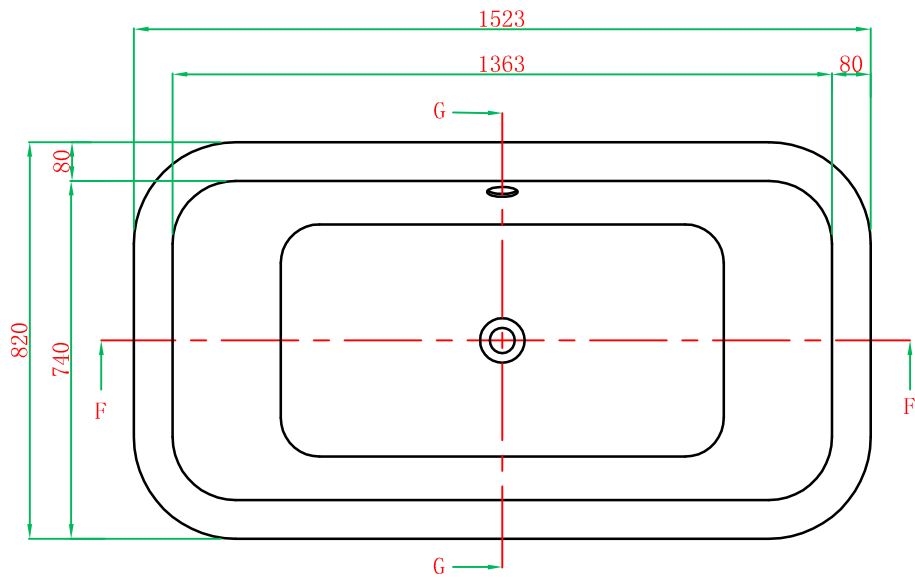
主视图
