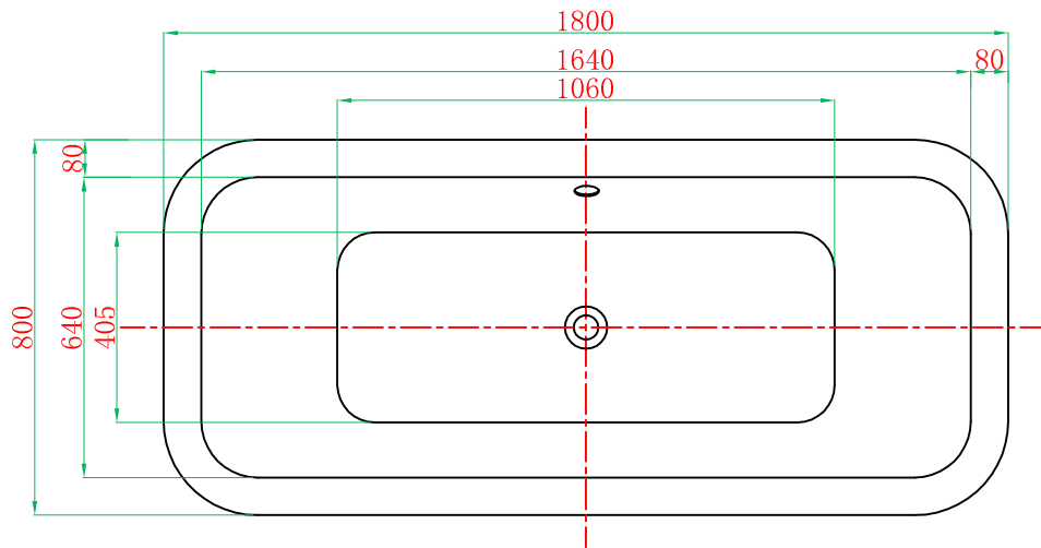
主视图
