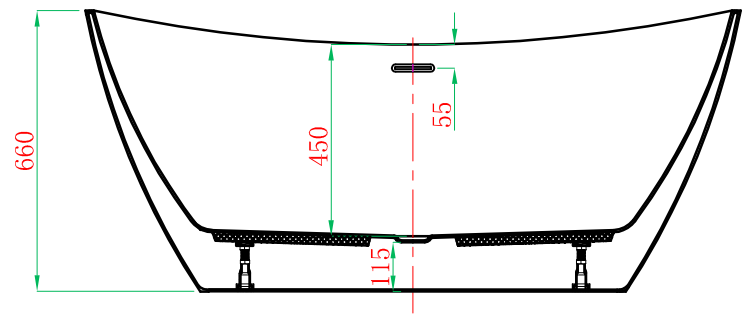
截面 F-F
