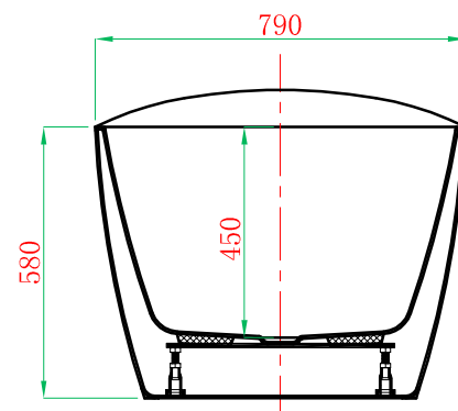
截面 G-G
