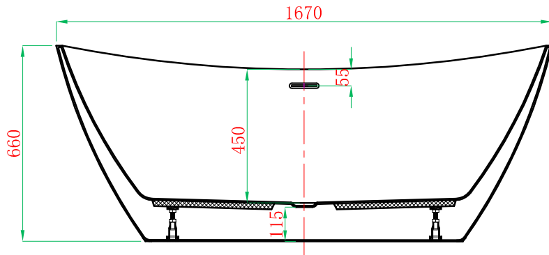
截面 F-F
