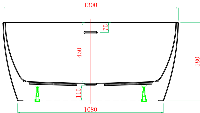
截面 F-F
