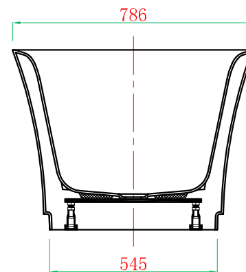
截面 G-G
